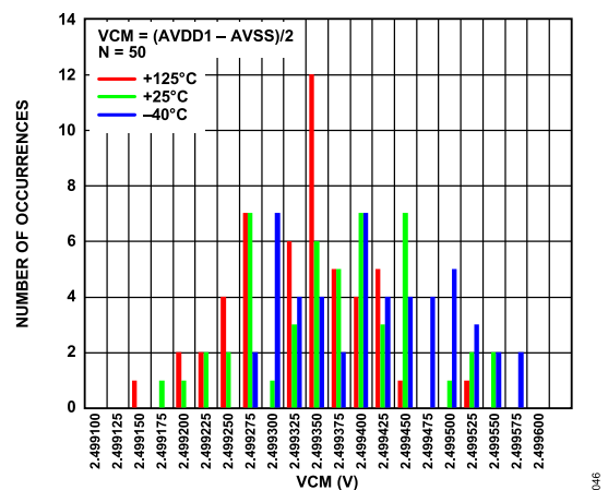
Figure 45. VCM Output Voltage Distribution, V_{CM} = (AVDD1 - AVSS)/2
